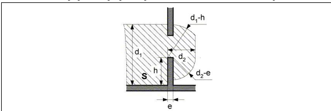
Abbildung 2.4 - Handbereich: Es gibt Öffnungen in den Ausrüstungselementen, die den Handbereich abgrenzen und den Durchgang eines langen geradlinigen Stabs von 12 mm Durchmesser nicht ermöglichen.
