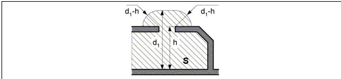
Abbildung 2.5 - Handbereich: Es gibt Öffnungen in den Ausrüstungselementen, die den Handbereich abgrenzen und den Durchgang eines langen geradlinigen Stabs von 12 mm Durchmesser nicht ermöglichen.
