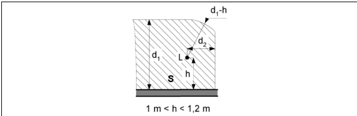
Abbildung 2.3 - Handbereich: Die Standfläche wird durch ein Ausrüstungselement abgegrenzt.
