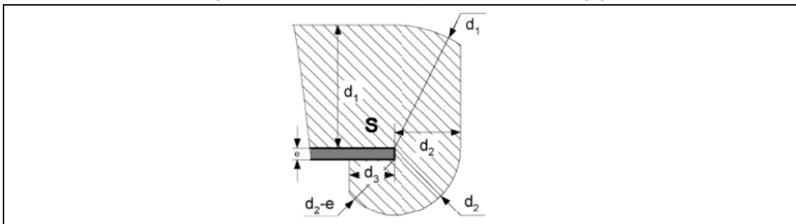
Abbildung 2.3 - Handbereich: Die Standfläche wird durch ein Ausrüstungselement abgegrenzt.
