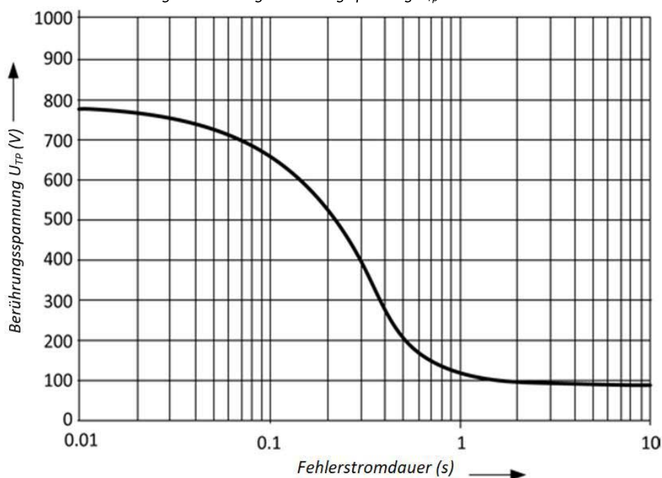
Abbildung 2.1 - Zulässige Berührungsspannung U_{Tp} im Verhältnis zur Fehlerstromdauer
