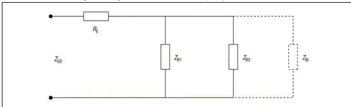
Abbildung 2.11 - Vergleichbares Schema der Schleifenimpedanz eines Erders Z_{EB}
