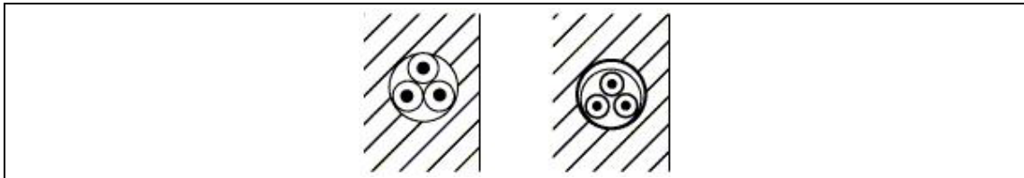
Abbildung 5.15 - Verlegearten für elektrische Leitungen - Aussparungen
