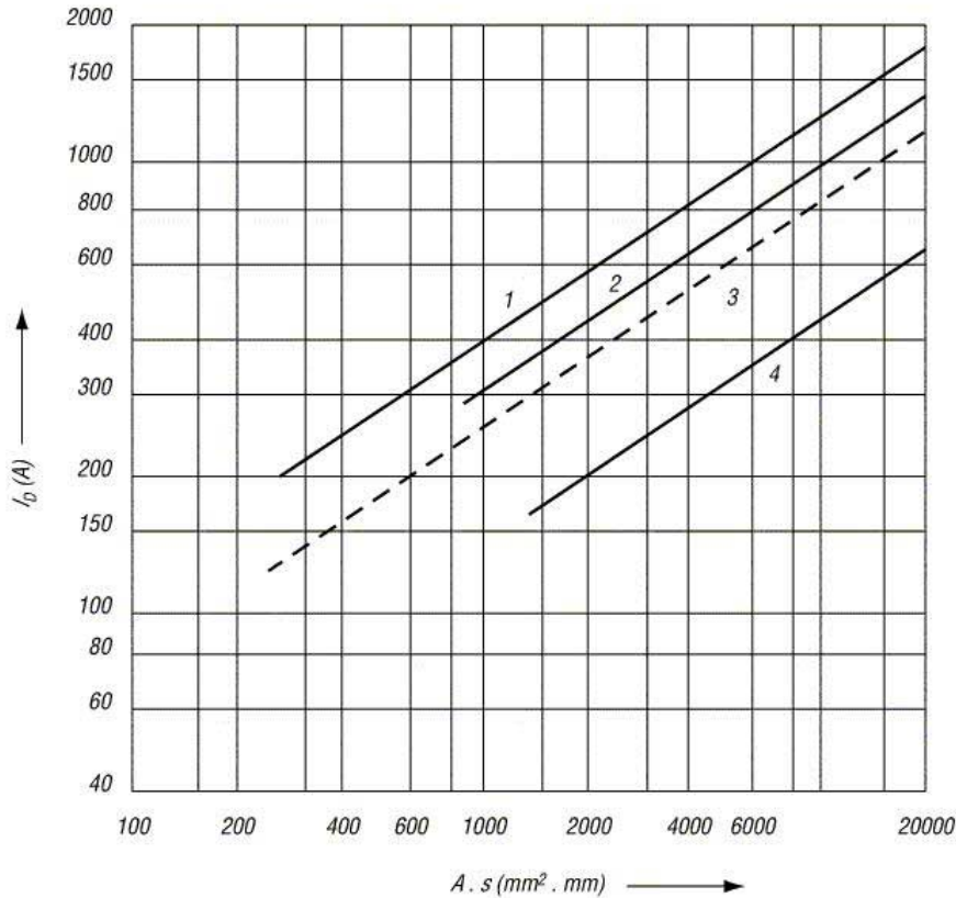
Abbildung 5.20 - Strom I_D für Erdungsleiter mit rechteckigem Querschnitt als Funktion der Produkts von Querschnitt und Umfang ( A \cdot s )
