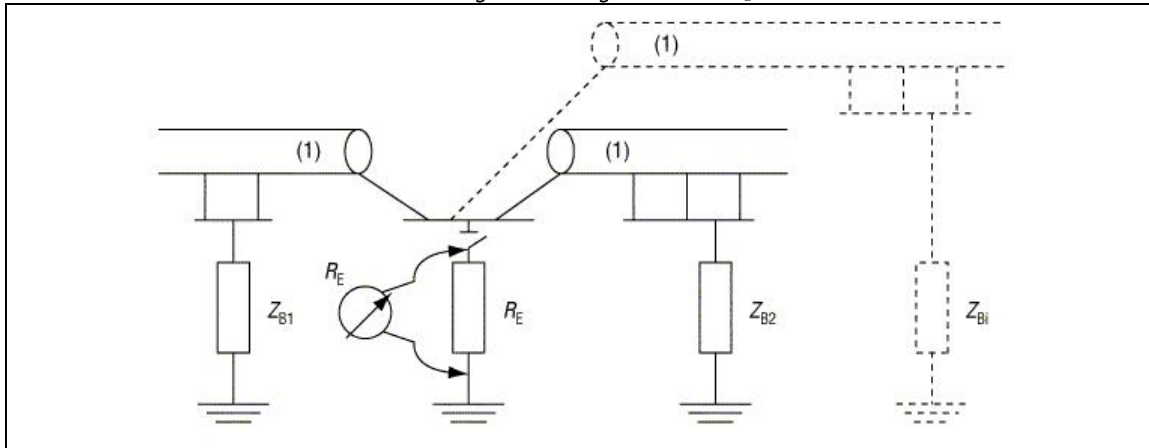
Abbildung 2.7 - Erdungswiderstand R_E
