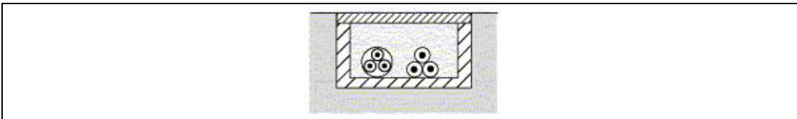
Abbildung 5.9 - Verlegearten für elektrische Leitungen - Direkte Verlegung in sandgefüllten Kabelkanälen
