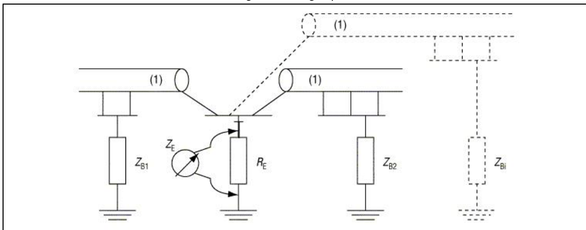
Abbildung 2.8 - Erdungsimpedanz Z_E
