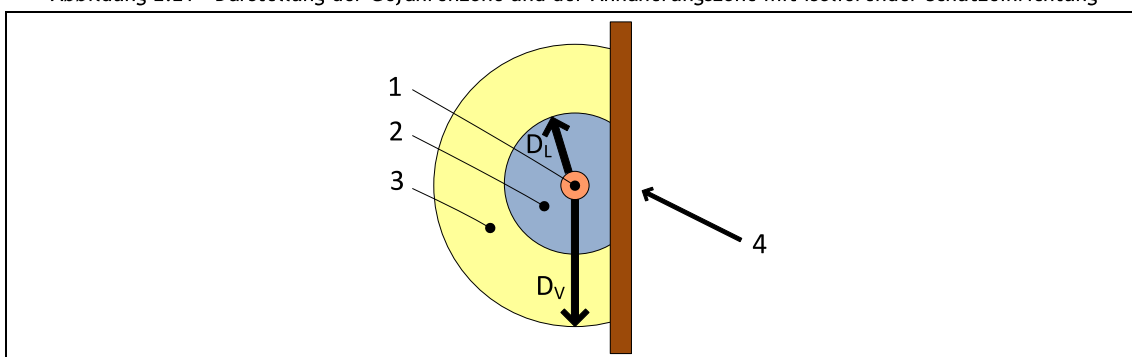
Abbildung 2.21 - Darstellung der Gefahrenzone und der Annäherungszone mit isolierender Schutzeinrichtung
