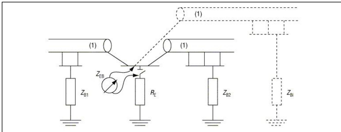
Abbildung 2.10 - Schleifenimpedanz eines Erders Z_{EB}
