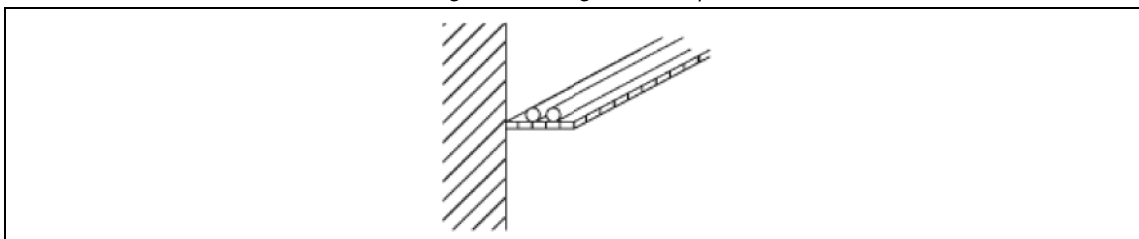
Abbildung 2.19 - Verlegeart "Kabelpritsche"
