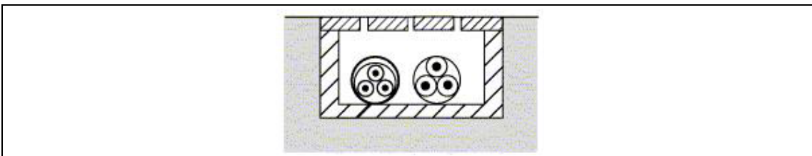
Abbildung 5.11 - Verlegearten für elektrische Leitungen - Elektroinstallationsrohre in offenen oder belüfteten Kabelkanälen
