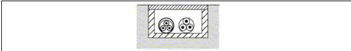
Abbildung 5.12 - Verlegearten für elektrische Leitungen - Elektroinstallationsrohre in geschlossenen Kabelkanälen
