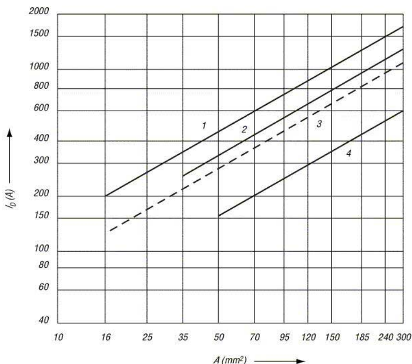
Abbildung 5.19 - Strom I_0 für Erdungsleiter mit kreisförmigem Querschnitt als Funktion ihres Querschnitts ( A in \text{mm}^2 )
