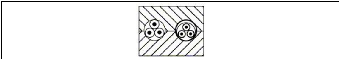
Abbildung 5.16 - Verlegearten für elektrische Leitungen - Vorgefertigte Blöcke
