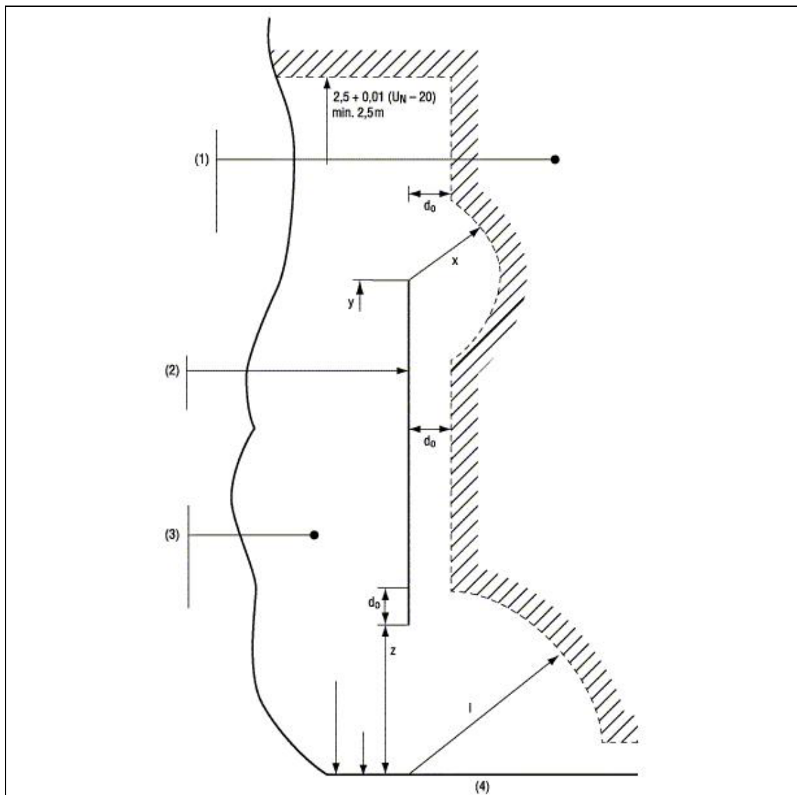
Abbildung 4.1 - Mindestabstände für den Schutz anhand von Hindernissen
