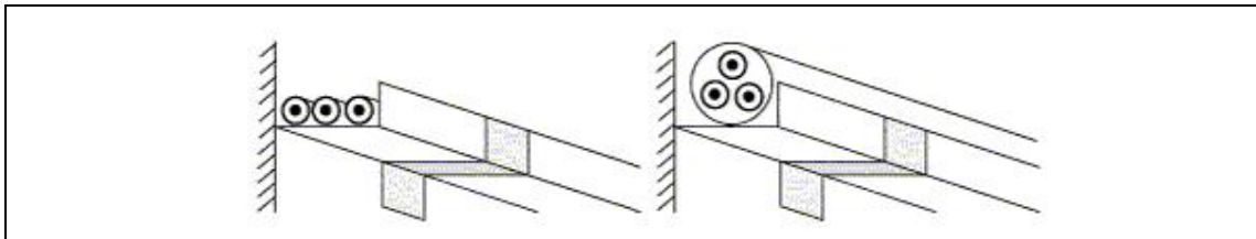
Abbildung 5.5 - Verlegearten für elektrische Leitungen - Kabelwannen
