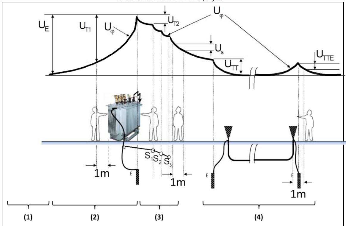
Abbildung 2.6 - Beispiel für die Veränderung des Erdoberflächenpotentials und der Spannungen, wenn Ströme durch die Erder fließen
