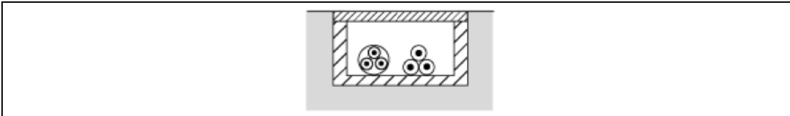
Abbildung 5.8 - Verlegearten für elektrische Leitungen - Direkte Verlegung in geschlossenen Kabelkanälen
