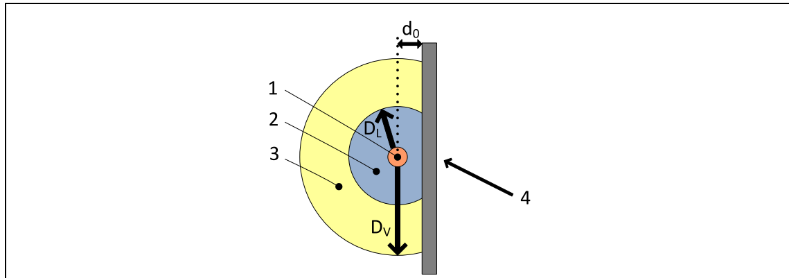
Abbildung 2.22 - Darstellung der Gefahrenzone und der Annäherungszone mit geerdeter metallischer Schutzeinrichtung
