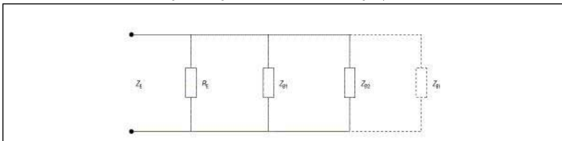
Abbildung 2.9 - Vergleichbares Schema der Erdungsimpedanz Z_E
