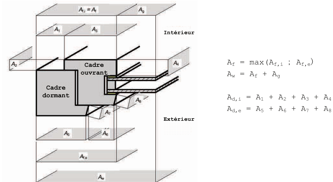
Figure [12] : Illustration des différentes surfaces
