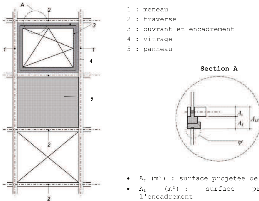
Figure [21] : Éléments constitutifs d'un mur rideau
