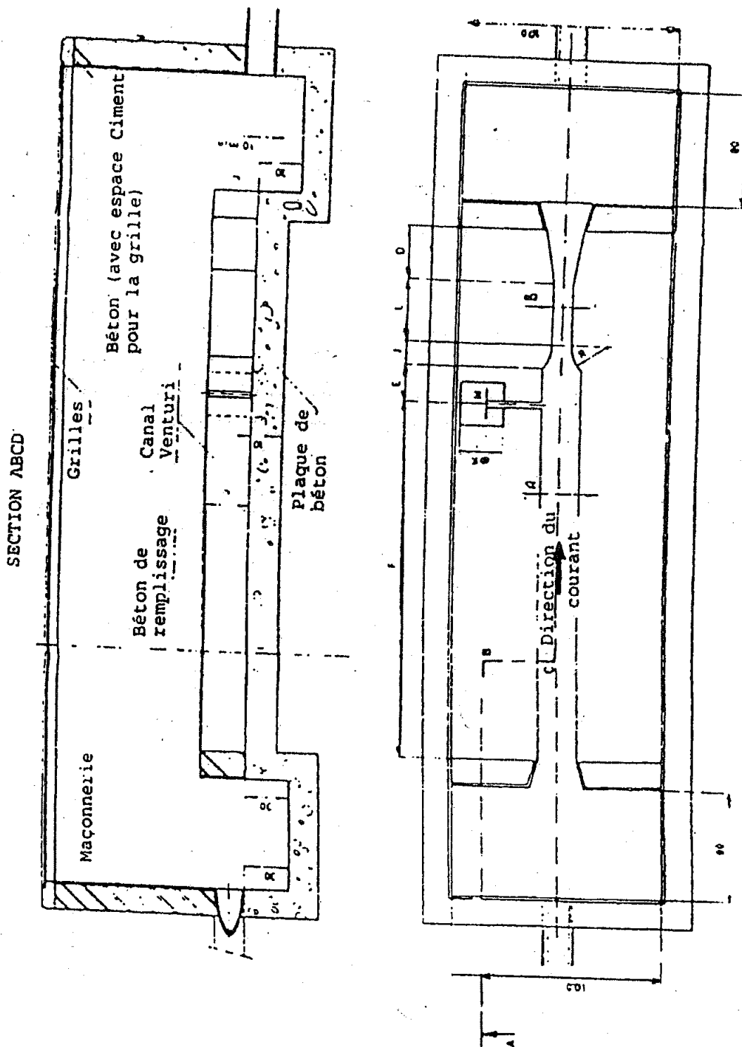
PLAN D'ENCASTREMENT DU CANIVEAU DE MESURE
