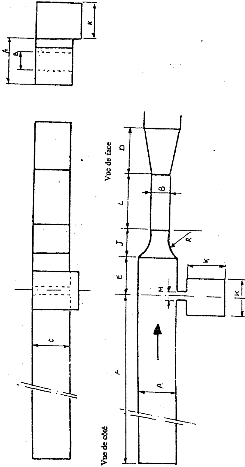
CANIVEAU DE MESURE A FOND PLAT.
